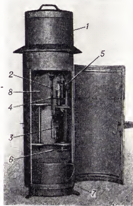
Рис. 1. Плювиограф.
